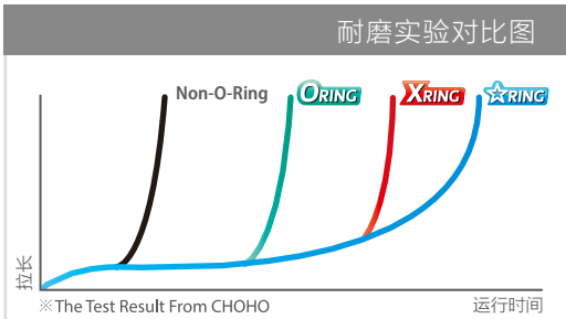
征和采用“星型”密封圈
