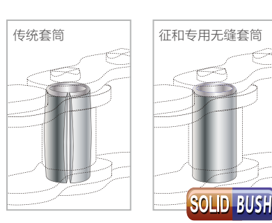
无缝套筒，采用冷挤压技术使用成型，圆筒无缝隙，圆筒无变形，真圆度大大提高，不易变形。无缝套筒与销轴的配合是以面接触而不是以点接触，增加产品耐磨性
