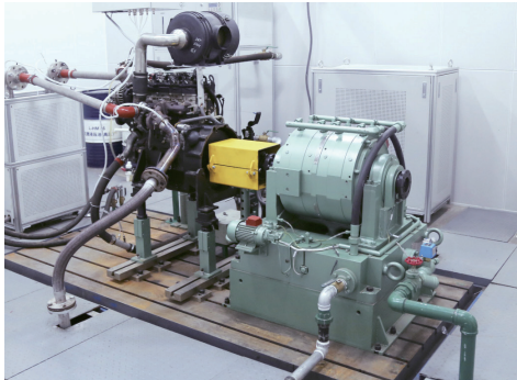
电涡流测功机试验台架系统 Eddy Current Dynamometer Test Bench System
