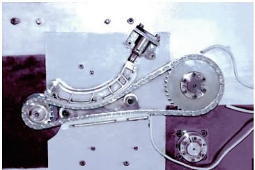
综合性能试验台 Comprehensive Performance Test Platform
